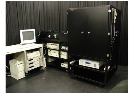
共同研究で利用した分光応答度標準校正装置
